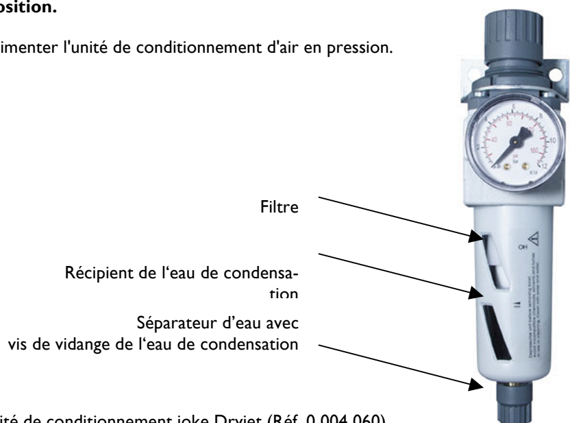
Fig. 9.1 Unité de conditionnement joke Dryjet (Réf. 0 004 060)
